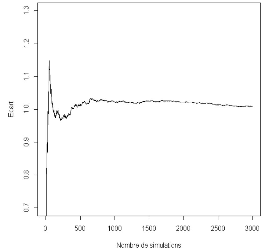
Ecart de convergence en fonction du nombre de simulations
